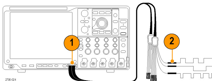
2790-024 Серии MSO5000B и DPO5000B
