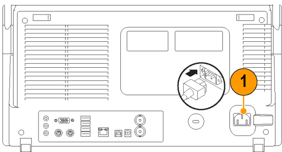
Серии MSO5000B и DPO5000B
