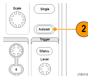
Серии MSO5000B и DPO5000B
